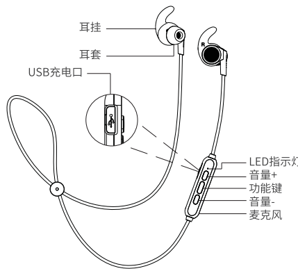
耳机示意图
